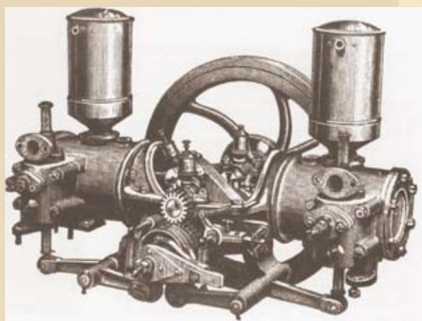
Nel 1895: Stabilimento Benz in Waldhofstrasse a Mannheim e il contra-motor
